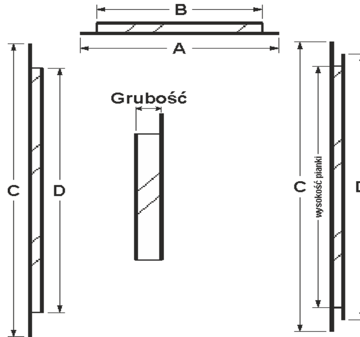
NAKŁADKA JEDNOSTRONNA
