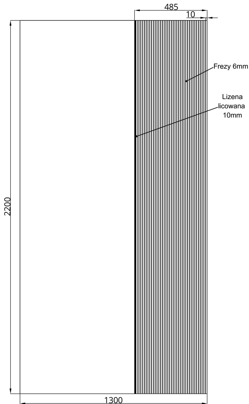
WIDOK OD STRONY ZEW.
