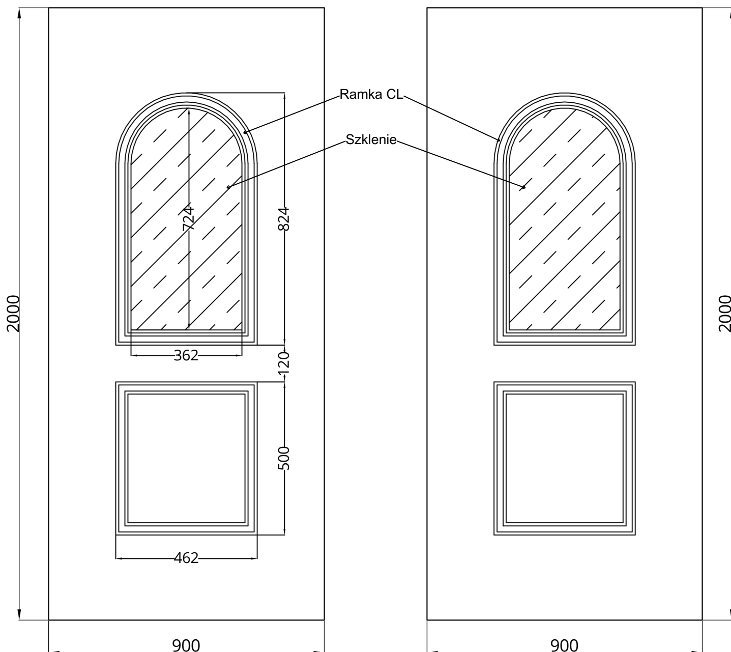
WIDOK OD STRONY ZEWN.
