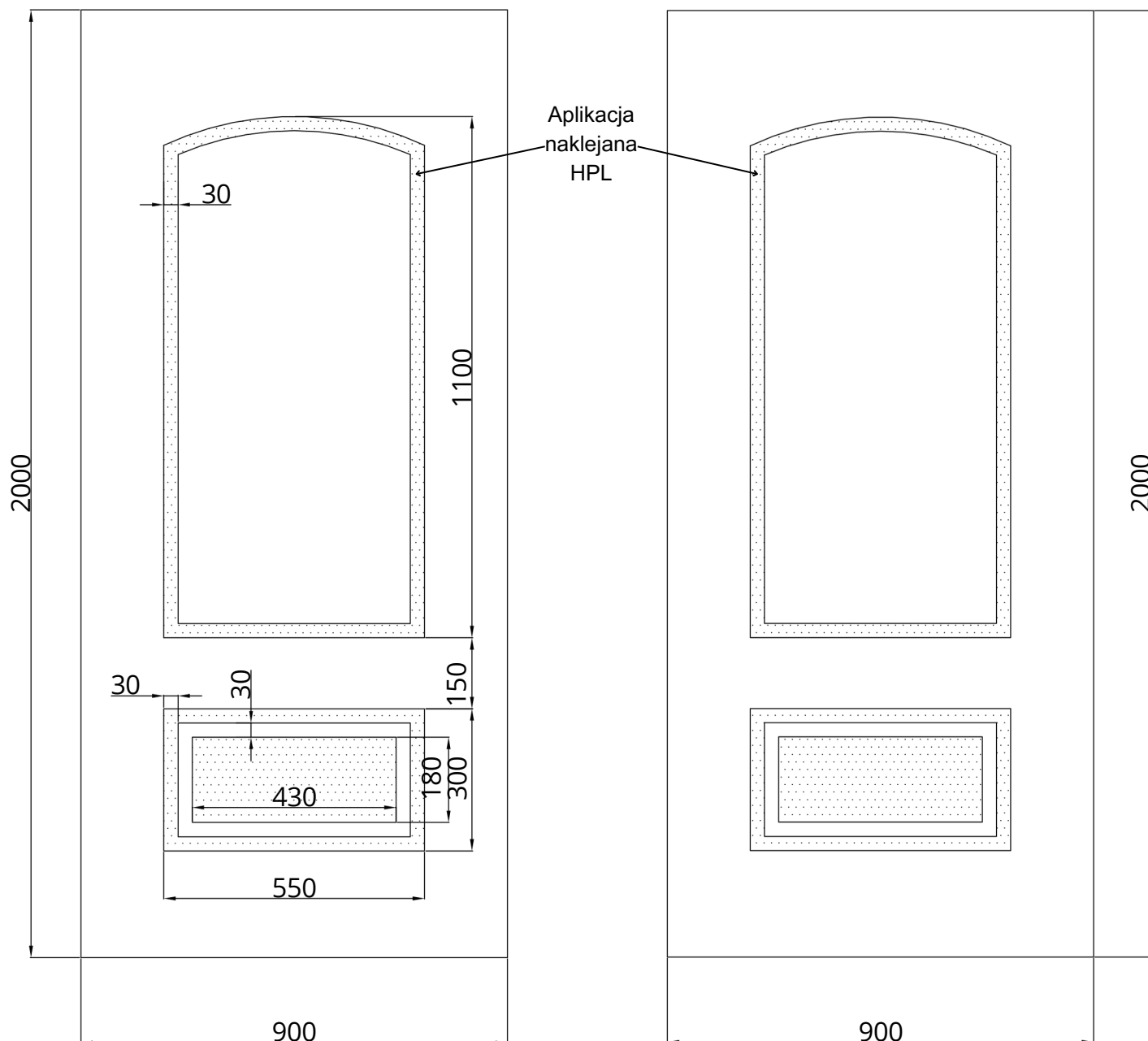
WIDOK OD STRONY ZEWN.
