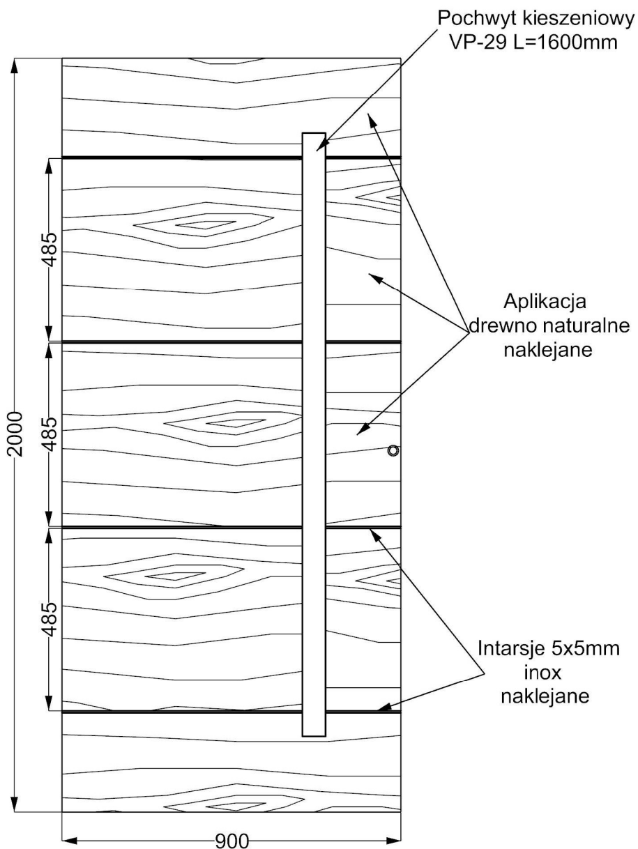
WIDOK OD STRONY ZEW.
